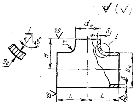
Переходный тройник
